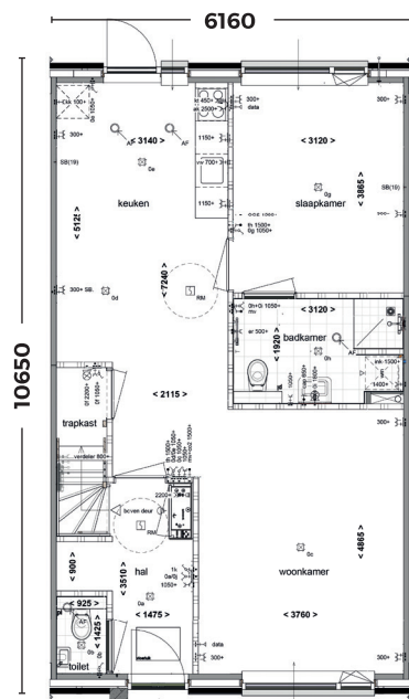
Begane grond
