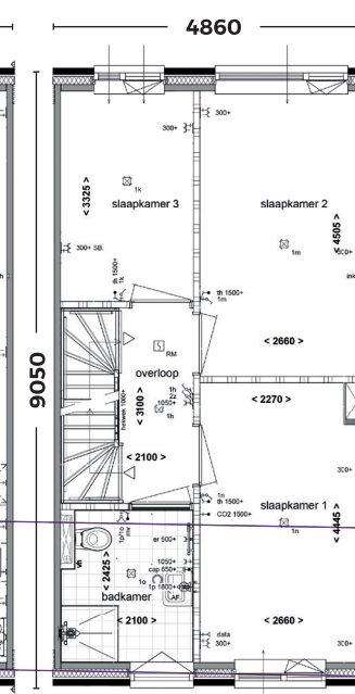
Eerste verdieping
