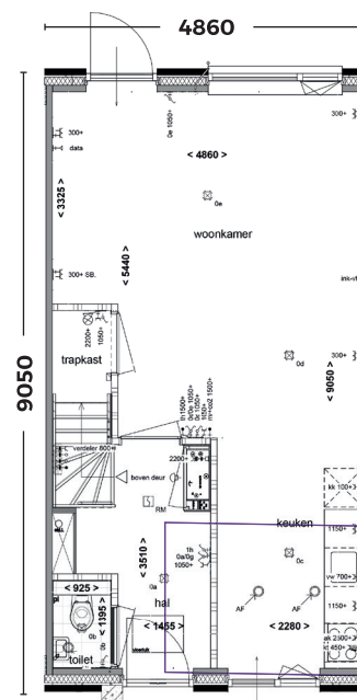
Begane grond
